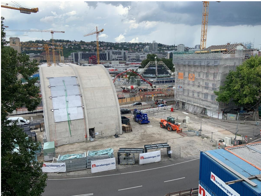
Abbildung 1: Blick auf das Baufeld bei Messbeginn am 14.08.2023
