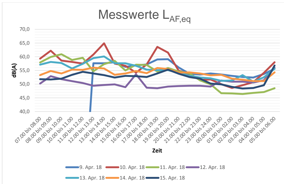
Bild 2: Pegelzeitverläufe für den Zeitraum vom 09.04.2018 bis 15.04.2018
