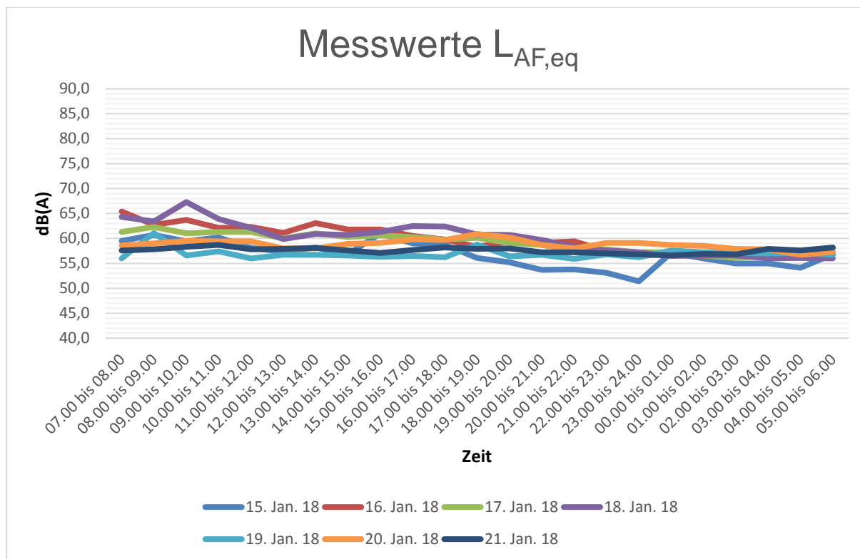
Bild 2: Pegelzeitverläufe für den Zeitraum vom 15.01.2018 bis 21.01.2018
