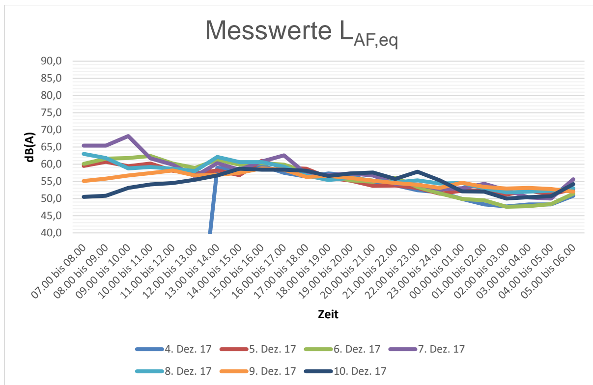
Bild 2: Pegelzeitverläufe für den Zeitraum vom 04.12.2017 bis 10.12.2017
