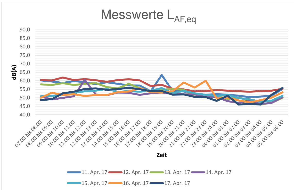
Bild 2: Pegelzeitverläufe für den Zeitraum vom 11.04.2017 bis 17.04.2017
