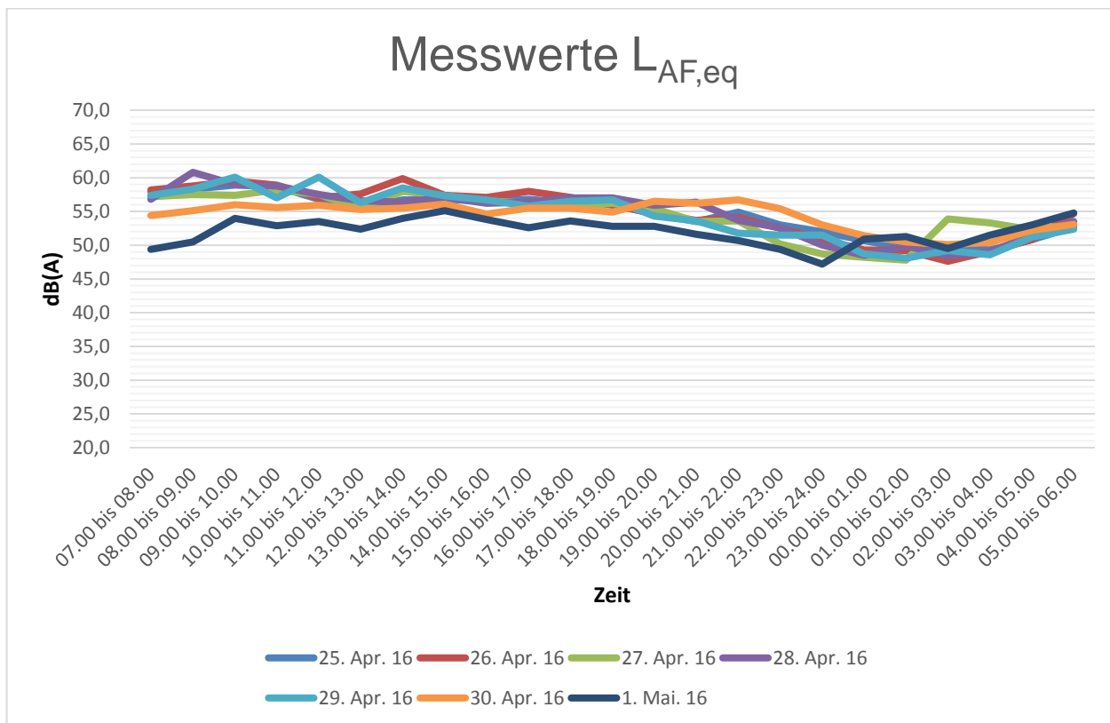
Bild 2: Pegelzeitverläufe für den Zeitraum vom 25.04.2016 bis 01.05.2016
